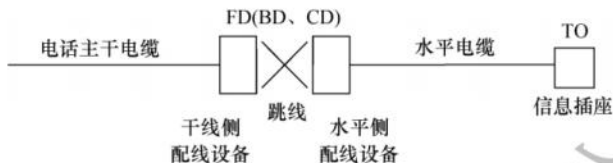
图 5.2.3-1 电话交换系统中缆线与配线设备间连接方式
