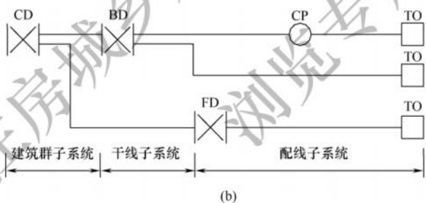
图 3.1.2-2 综合布线子系统构成
