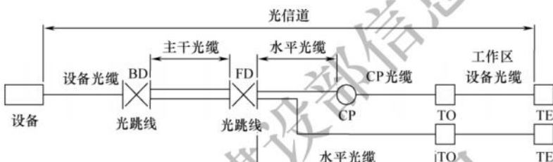
图 3.2.4-1 光纤信道构成 1
