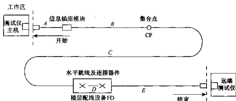
图 B.0.1-2 信道方式
