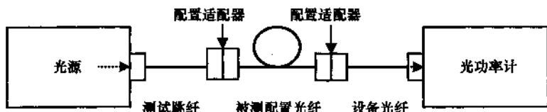
图3 单跳线信道测试连接方式
